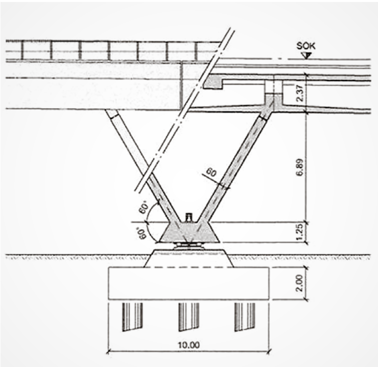
Ansicht und Querschnitt V-förmige Stützen
