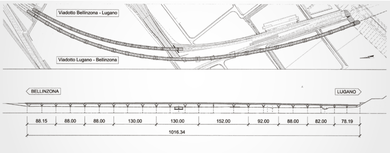
Situation + Längsschnitt Viadotto Bellinzona-Lugano und Viadotto Lugano-Bellinzona
